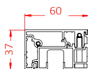
Z2 - Smal styrskena
