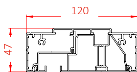
Z1 - Standard styrskena
