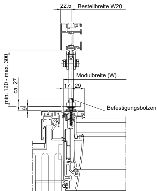
Schnitt A-A: Einzelführungsschiene
