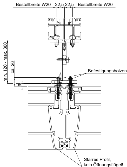
Schnitt A-A: Doppelführungsschiene
