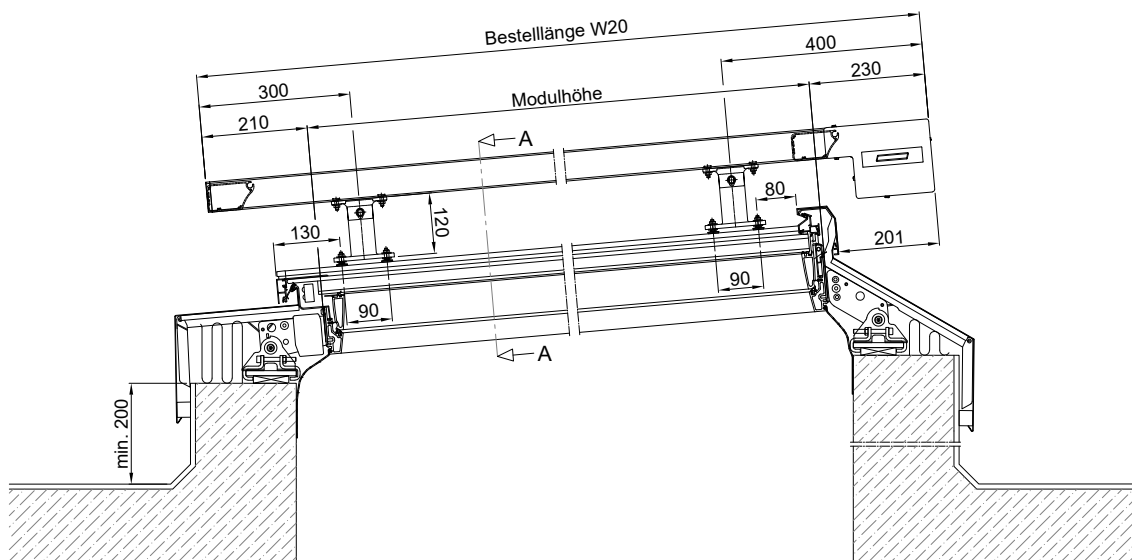
Wintergarten-Markise Climara W20 mit eckiger Blende
