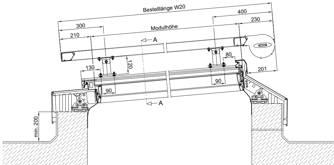
Wintergarten-Markise Climara W20 mit runder Blende
