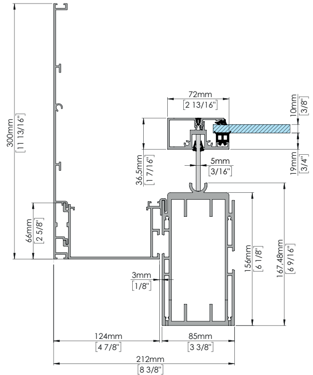
Bezeichnung: Vertikalschnitt, Randsparren mit Füllung
