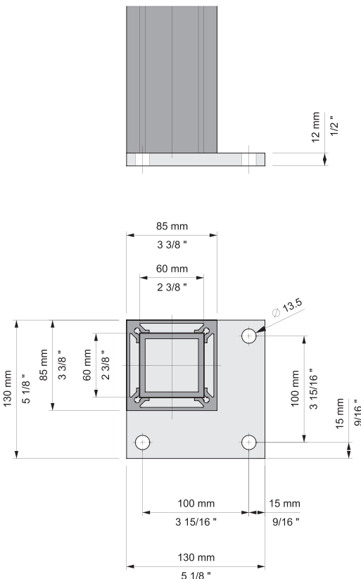
Bezeichnung: Schnitt, Stütze mit Stützfuß Ecke
