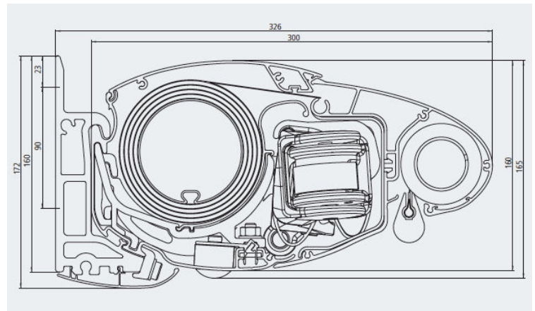
Vægmontage (loftsmontage også muligt med andre beslag)
