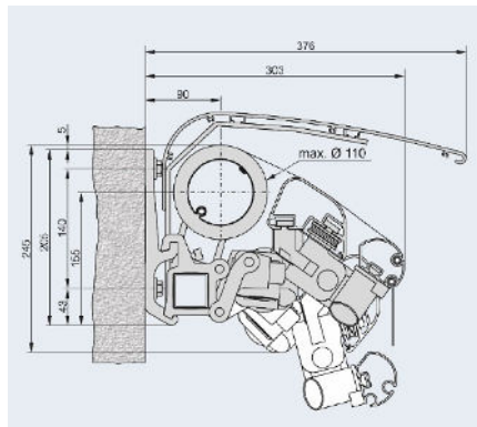
Snittegning standard loftmontage
