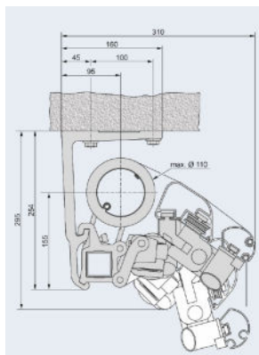
Snittegning standard loftmontage
