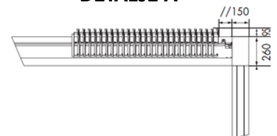
DETALJE A
