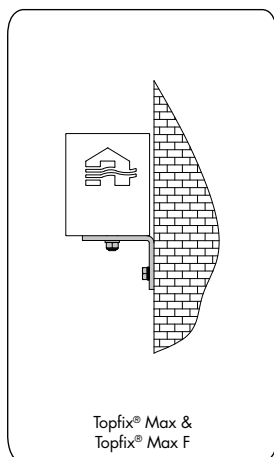
Wandbefestigung der Seitenführungen
