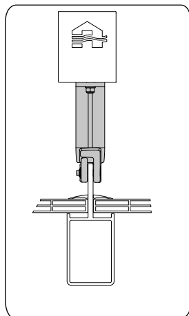
Befestigung der Montagefüße bei einem T-Träger (darunter liegendes Glas)
