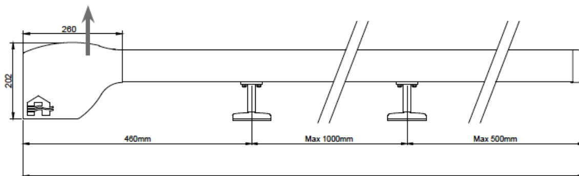
Snit fra siden
