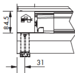
Snit fra front
