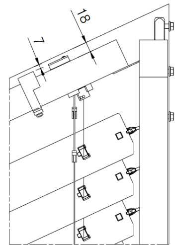
Lameldetaljer i top
