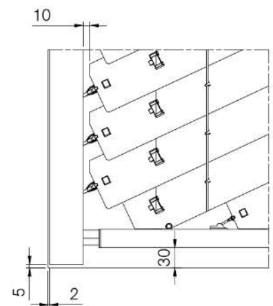
Lameldetaljer i bund
